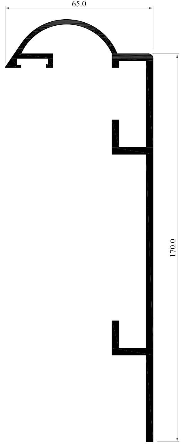
794 Kasa Dış Profili
