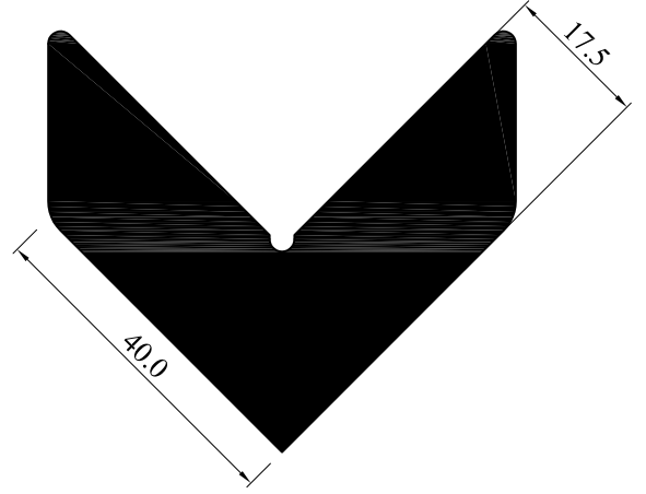
C90-175 Çavuş Gönye
