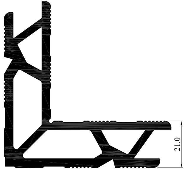
T851-210 Köşe Takoğu ( 54031-12 de kullanılır )
