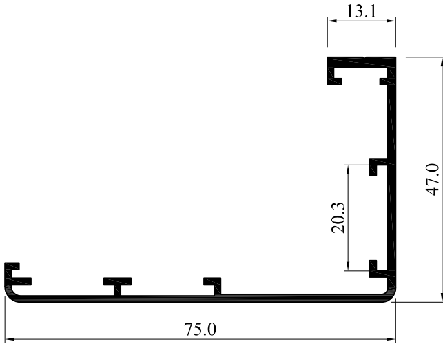
54051-15 Kasa Dış Profili ( 85-110mm )
