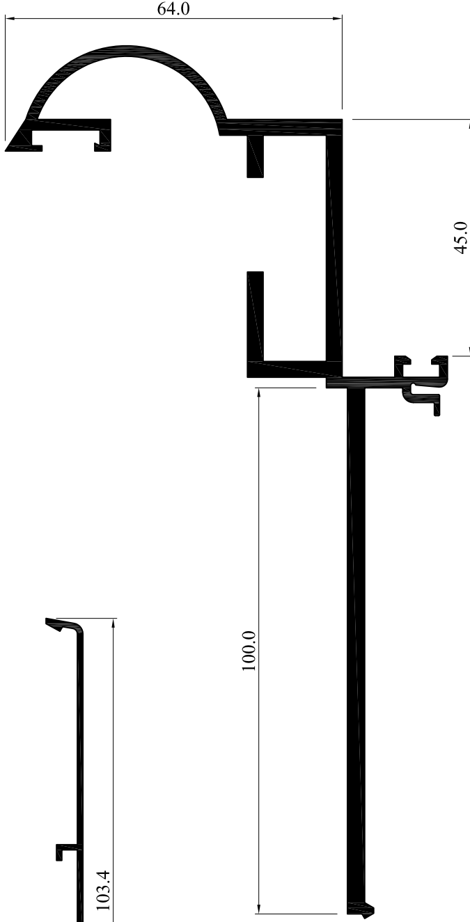
793 Kasa İç Profili
