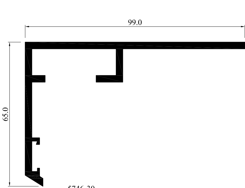
5746-30 Kasa Dış Profili
