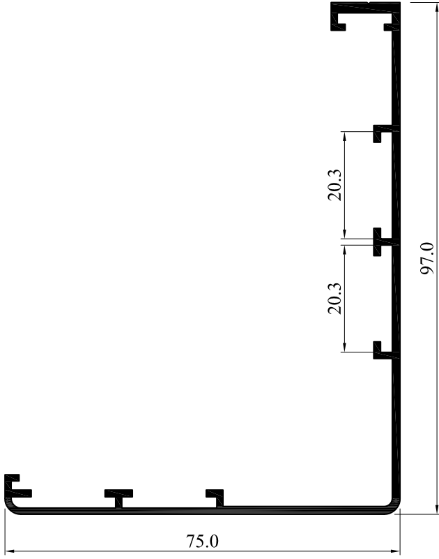
54053-15 Kasa Dış Profili ( 135-160mm )
