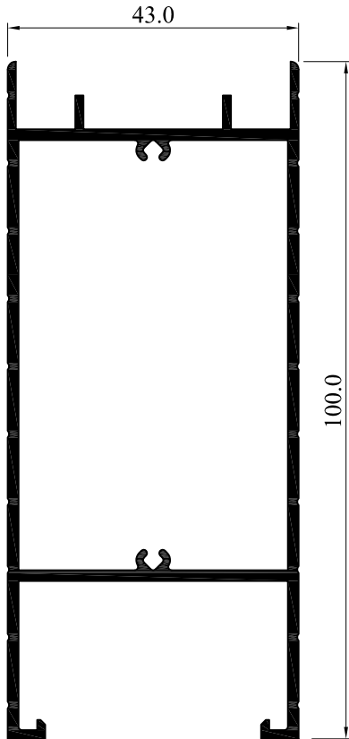
54053-15 Kasa Dış Profili ( 135-160mm )
