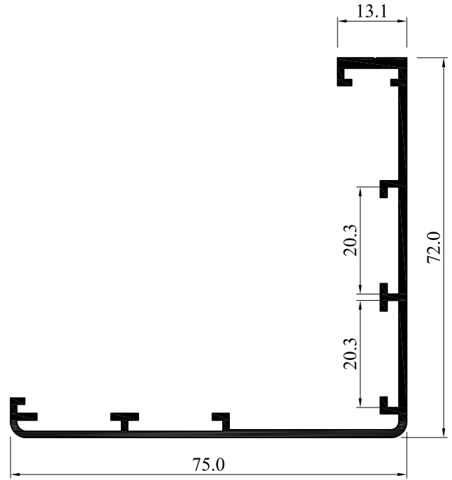
54052-15 Kasa Dış Profili ( 110-135mm )
