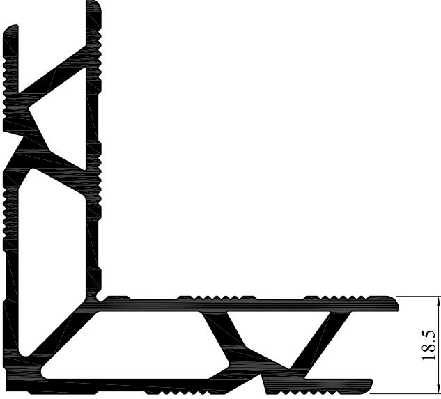
T851-185 Köşe Takoğu ( 54011-15 de kullanılır )
