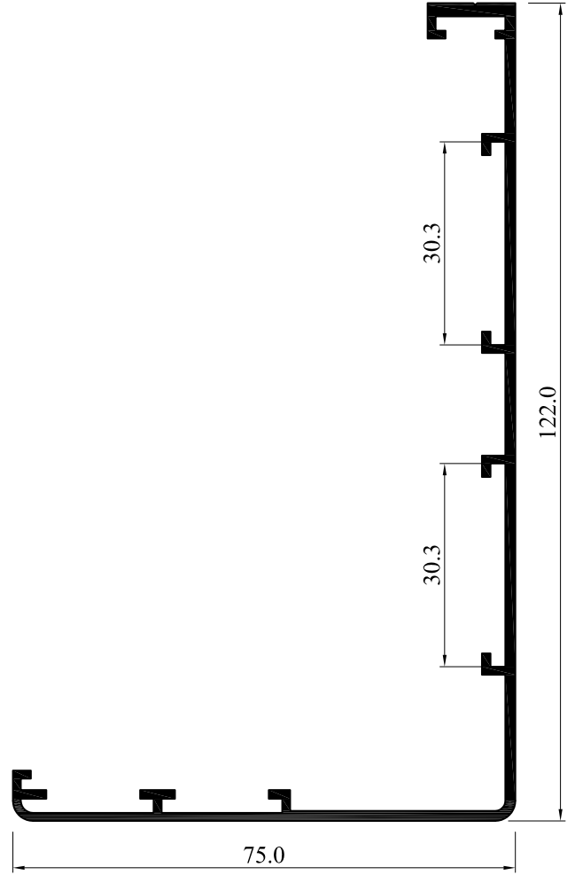
54054-15 Kasa Dış Profili ( 160-185mm )
